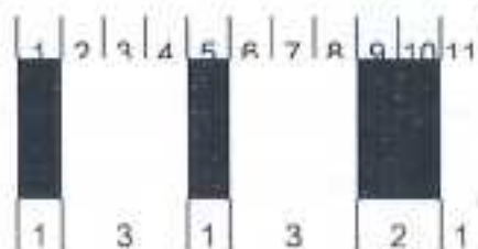
Hình 12 – Ký tự mã vạch giá trị 35 của mã vạch 128
