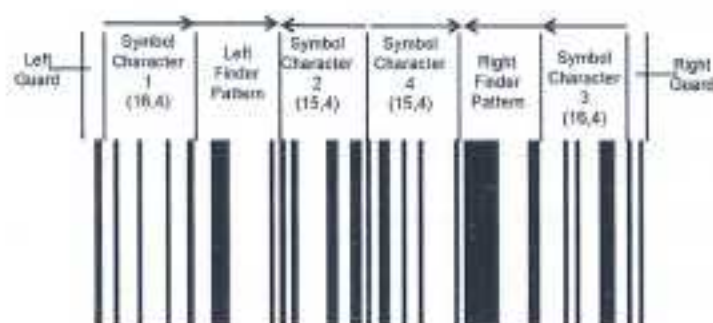
Hình 14 – Cấu trúc
